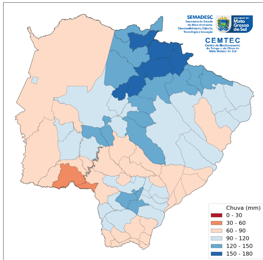
Figura 02 – Precipitação acumulada
