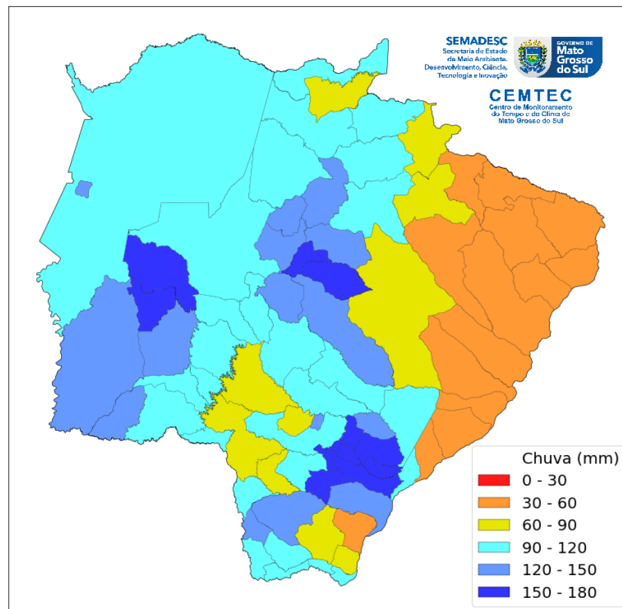
Figura 03 – Precipitação acumulada
