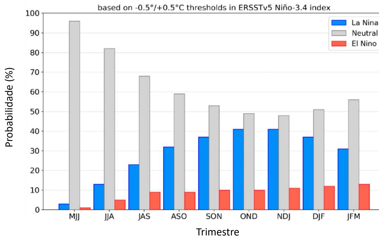
Gráfico 10 - Previsão probabilística do El Niño Oscilação Sul (ENOS) trimestral
