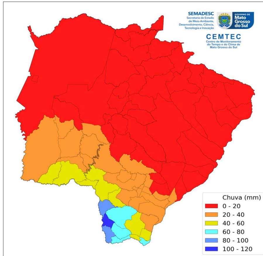
Figura 03 – Precipitação acumulada
