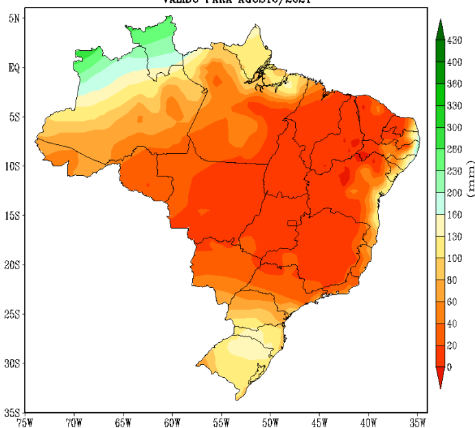
PRECIPITAÇÃO TOTAL PREVISTA (mm) ATUALIZAÇÃO - JULHO/2021 VÁLIDO PARA AGOSTO/2021
