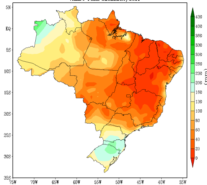
PRECIPITAÇÃO TOTAL PREVISTA (mm) ATUALIZAÇÃO - JULHO/2021 VÁLIDO PARA SETEMBRO/2021
