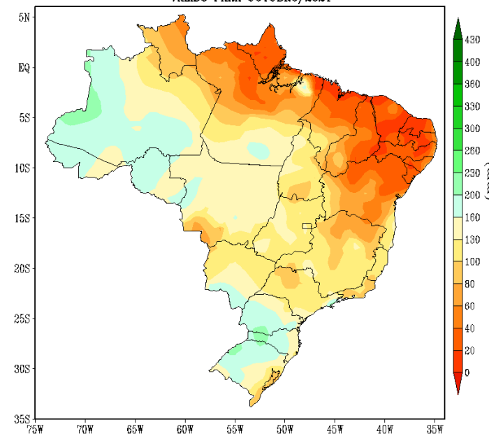
PRECIPITAÇÃO TOTAL PREVISTA (mm) ATUALIZAÇÃO - JULHO/2021 VÁLIDO PARA OUTUBRO/2021
