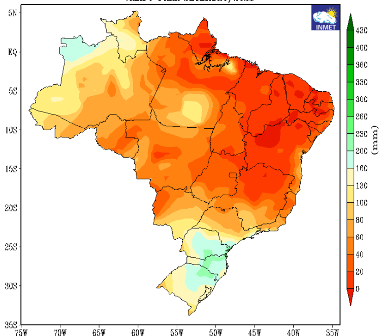
PRECIPITAÇÃO TOTAL PREVISTA (mm) ATUALIZAÇÃO - JULHO/2023 VALIDO PARA SETEMBRO/2023
