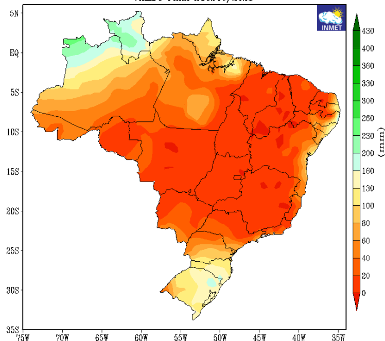
PRECIPITAÇÃO TOTAL PREVISTA (mm) ATUALIZAÇÃO - JULHO/2023 VALIDO PARA AGOSTO/2023
