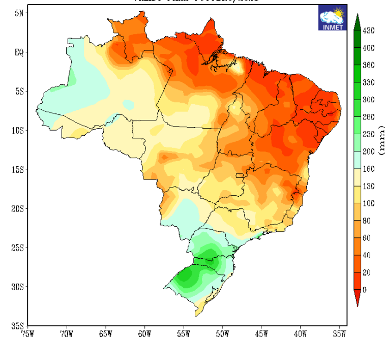
PRECIPITAÇÃO TOTAL PREVISTA (mm) ATUALIZAÇÃO - JULHO/2023 VALIDO PARA OUTUBRO/2023
