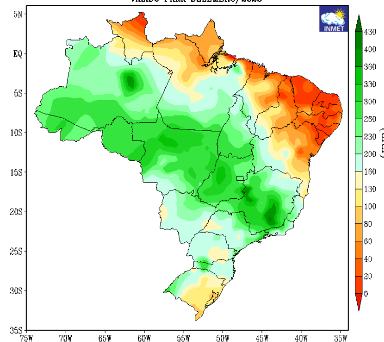
PRECIPITAÇÃO TOTAL PREVISTA (mm) ATUALIZAÇÃO - SETEMBRO/2023 VALIDO PARA DEZEMBRO/2023
