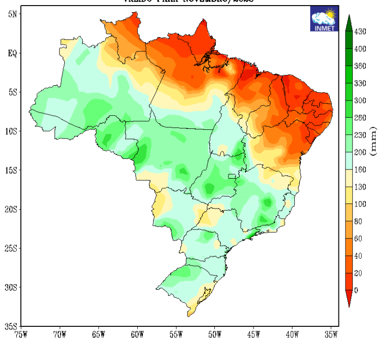
PRECIPITAÇÃO TOTAL PREVISTA (mm) ATUALIZAÇÃO - SETEMBRO/2023 VALIDO PARA NOVEMBRO/2023
