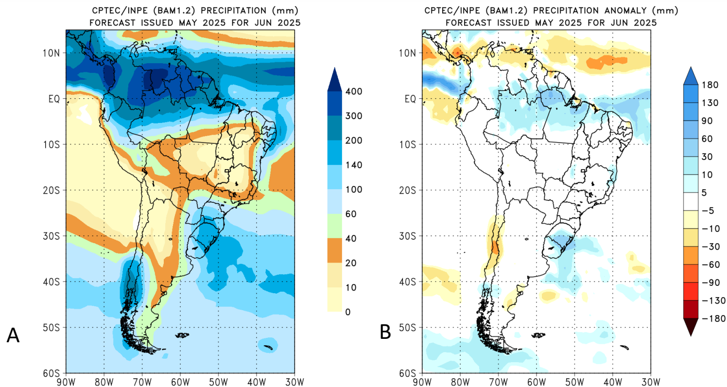
Figura 4. Prognóstico (a) e anomalia (b) da precipitação para o mês de Junho de 2025. Fonte: CPTEC/INPE.
