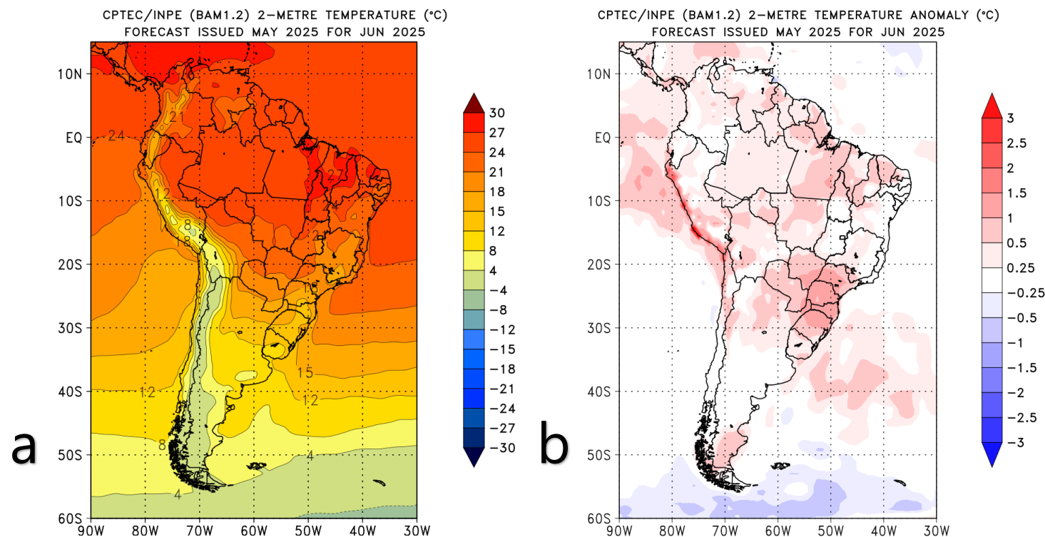
Figura 5. Prognóstico (a) e anomalia (b) da temperatura do ar para o mês de Junho de 2025. Fonte: CPTEC/INPE.
