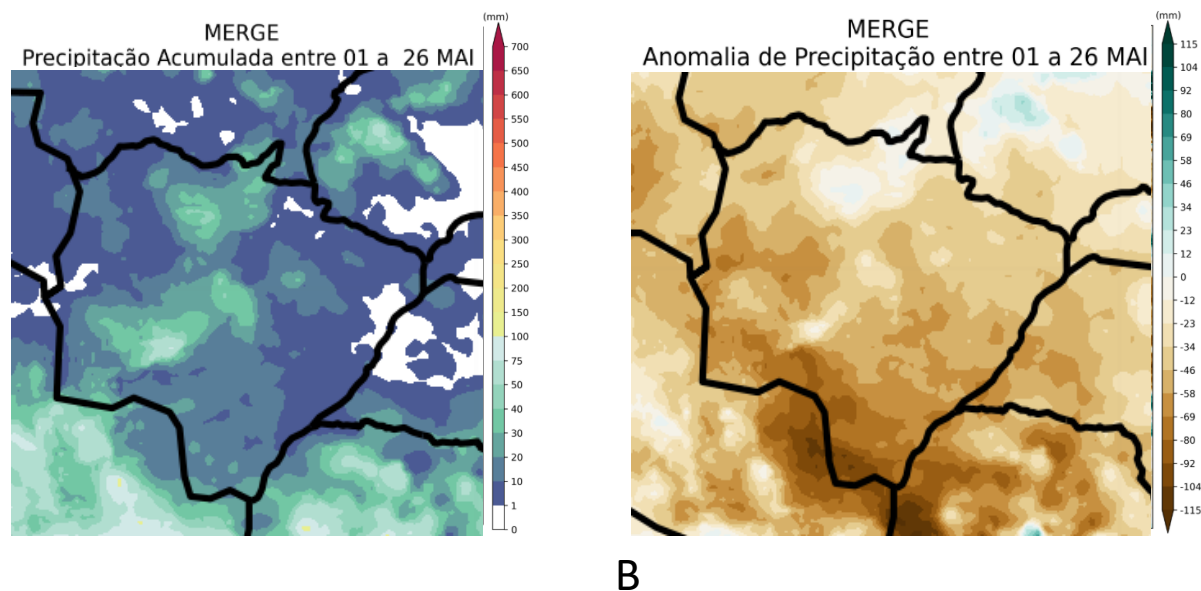
Figura 3. Precipitação acumulada (A) anomalia de precipitação (B) no estado de Mato Grosso do Sul entre 01 e 26 de maio de 2025. Fonte: Adaptado de MERGE/INPE/CPTEC.
