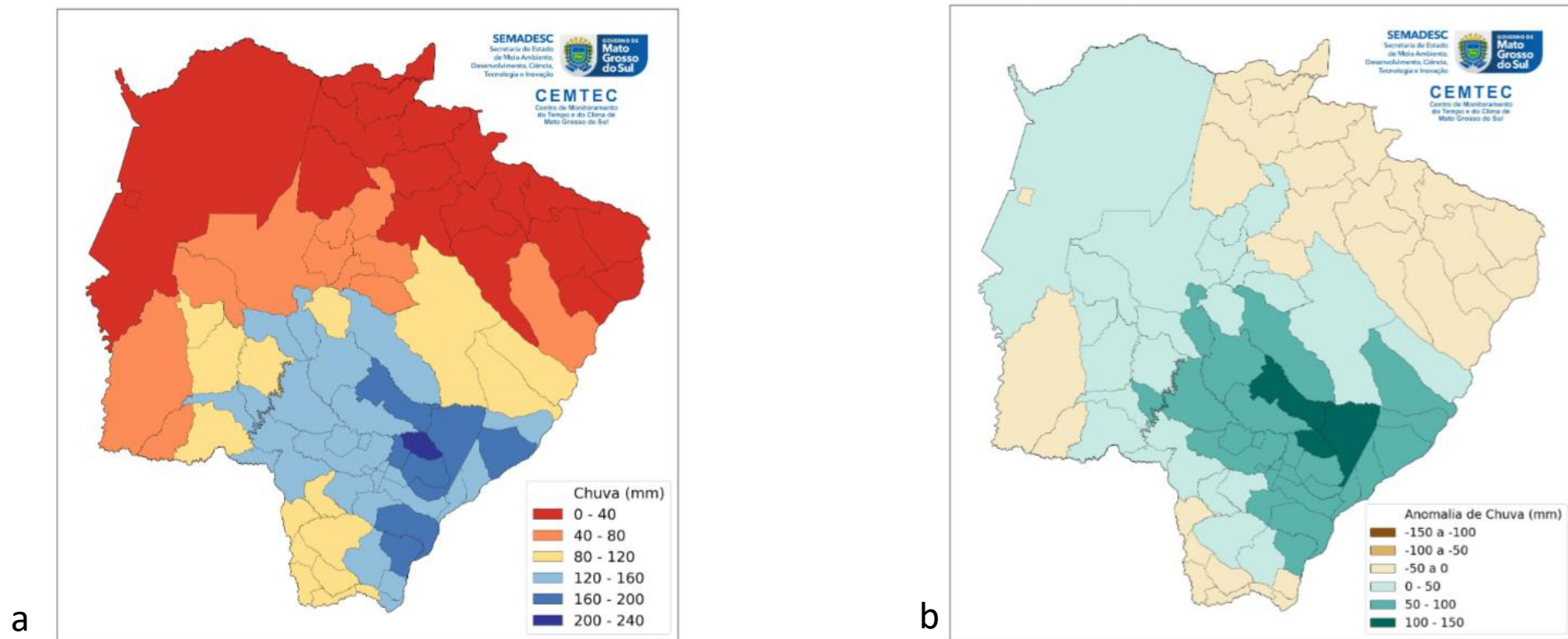
Figura 3. Precipitação acumulada durante o mês de maio de 2026 (a); Volume de chuva em relação à média histórica (b). Fonte dos dados: MERGE/INPE. Processamento de dados: CEMTEC.
