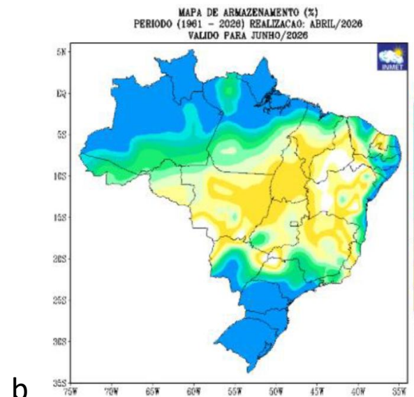
Figura 4. Nível de armazenamento de água no solo de municípios de Mato Grosso do Sul durante o mês de maio de 2026 (a); Prognóstico de armazenamento de água no solo para o mês de junho/26 (b). Fonte dos dados: a) INMET/SISDAGRO; b) boletim agro meteorológico edição abril/2026.
